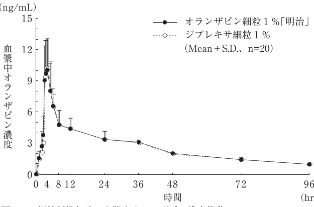
図5 1%細粒剤投与時の血漿中オランザピン濃度推移
