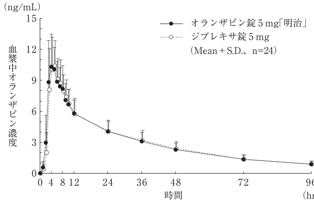
図2 5mg錠投与時の血漿中オランザピン濃度推移 表3 薬物動態パラメータ
